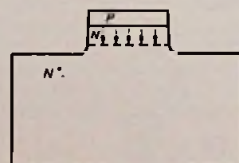
Fig. 6b. Mesa afstemdiode.
